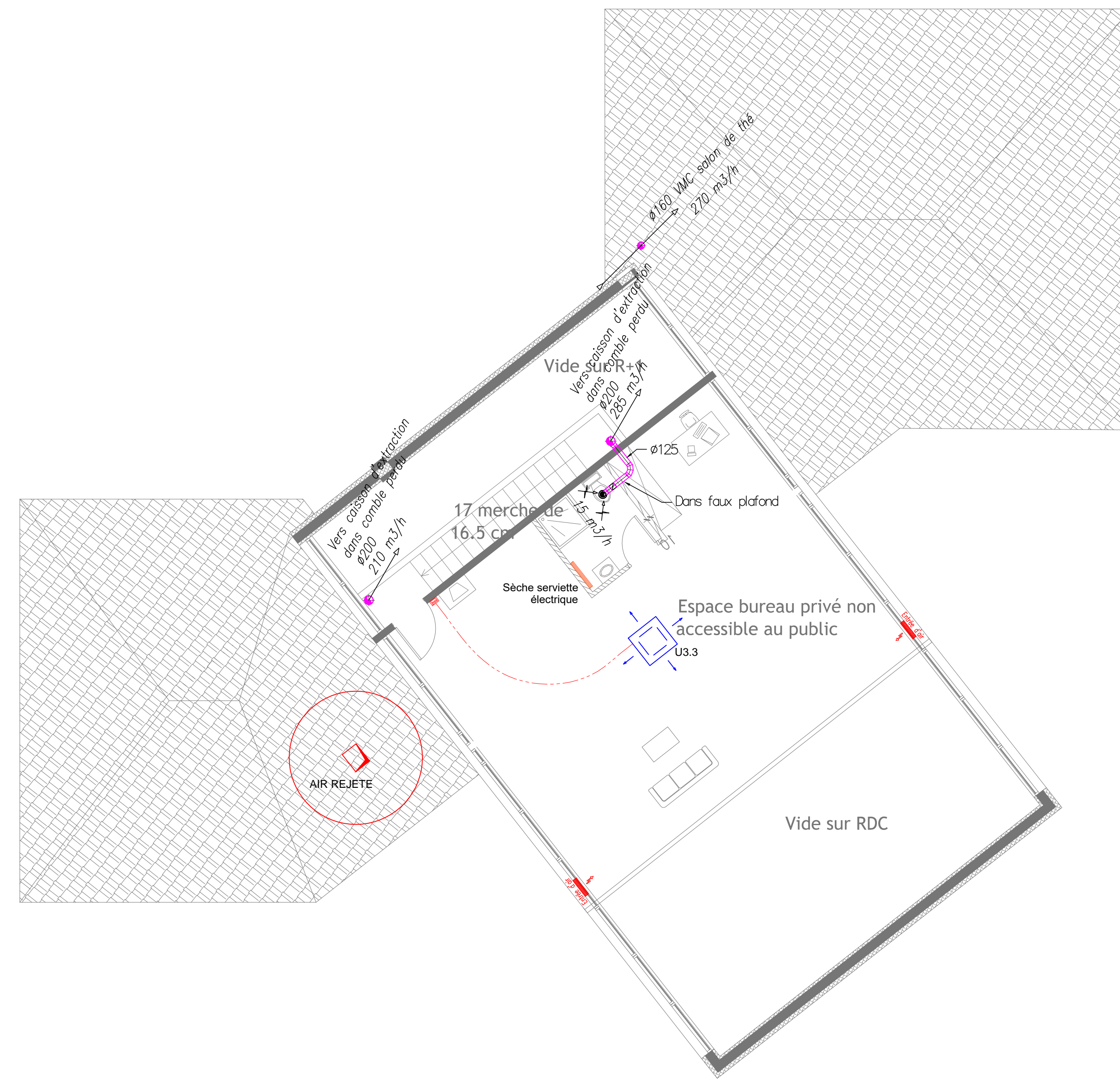
PLAN R+2
